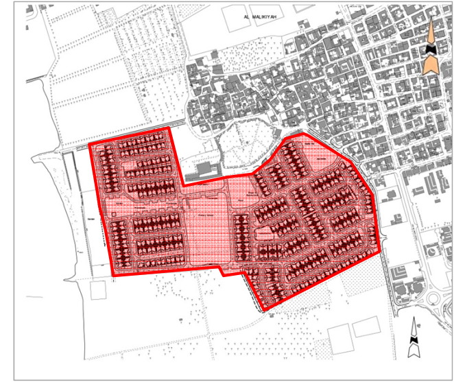
الموقع العام
