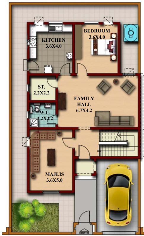
الطابق الأرضي
